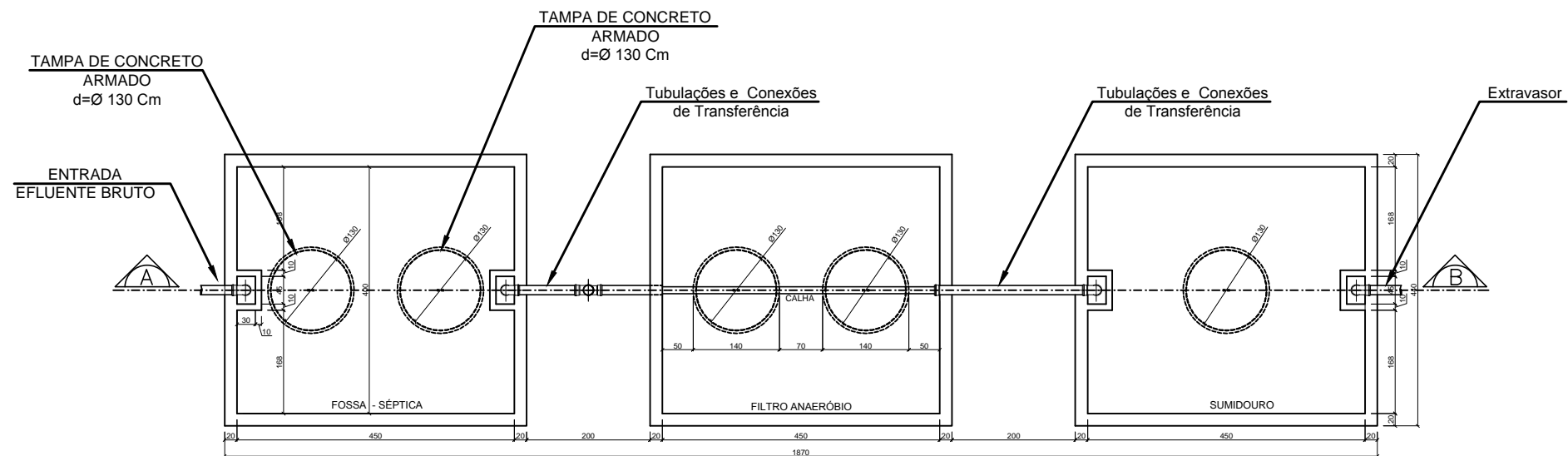
PLANTA BAIXA - SISTEMA FOSSA / FILTRO / SUMIDOURO
