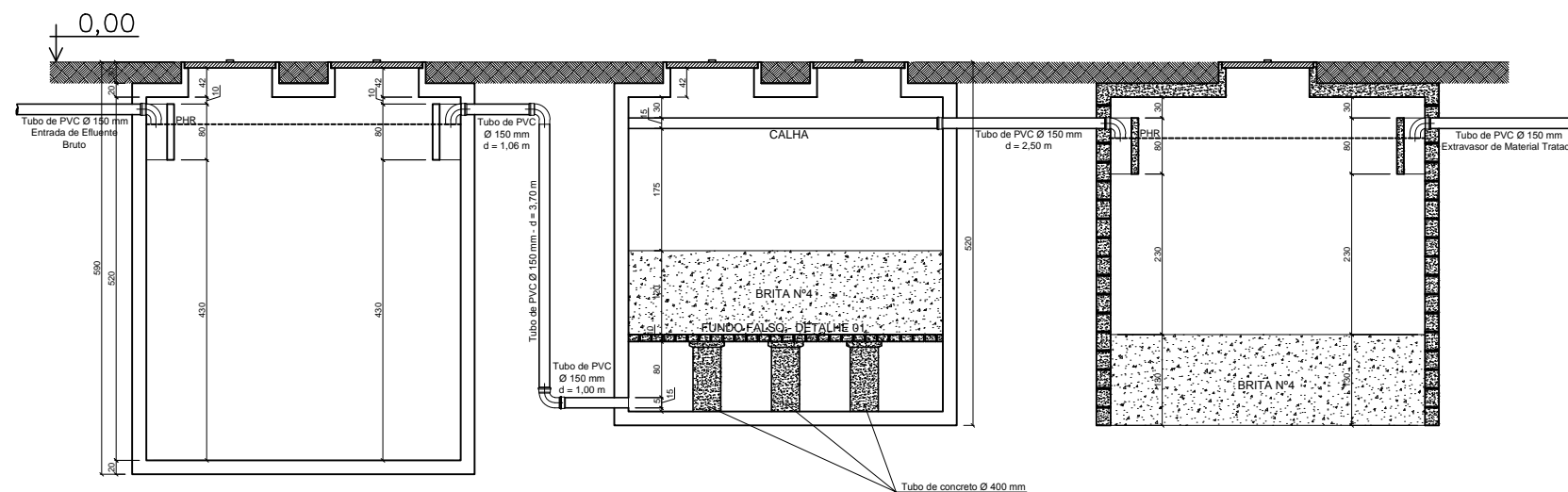
CORTE AB - SISTEMA FOSSA / FILTRO / SUMIDOURO
